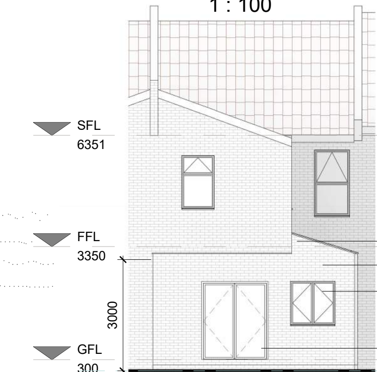
REAR 1 : 100
