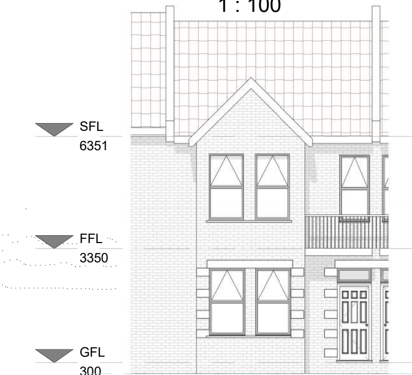
FRONT 1 : 100
