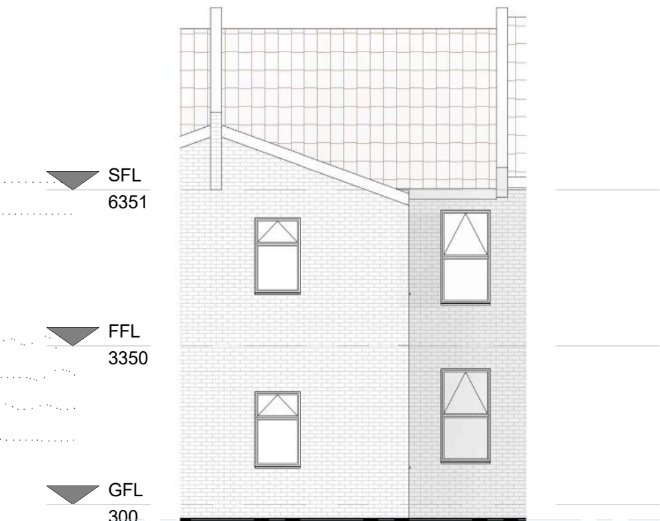
REAR 1 : 100
