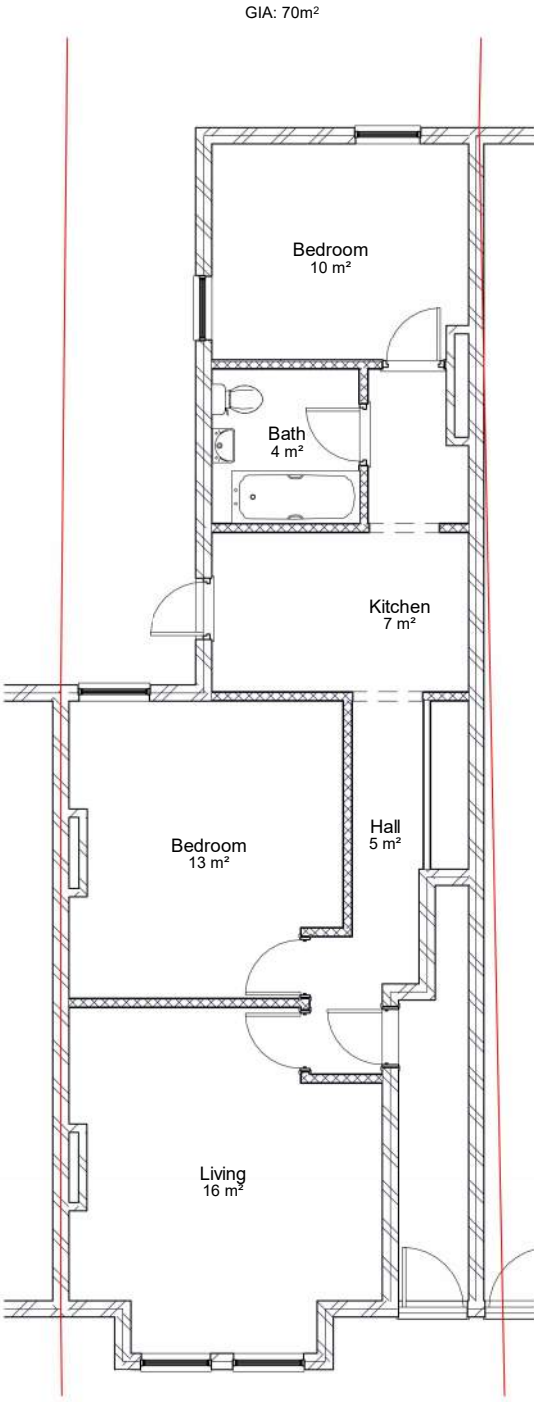
GFL 1 : 100
